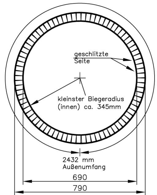
ELEMENT-EL SL/SQ 50
