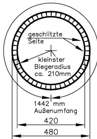
ELEMENT-EL SL/SQ 30
