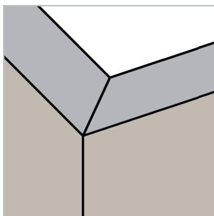
Hoeken verlijmd in de fabriek
