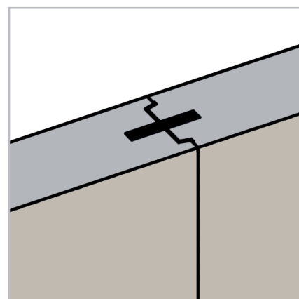
Paneelverbinding met groef en veer verbinding en V-inkeping
