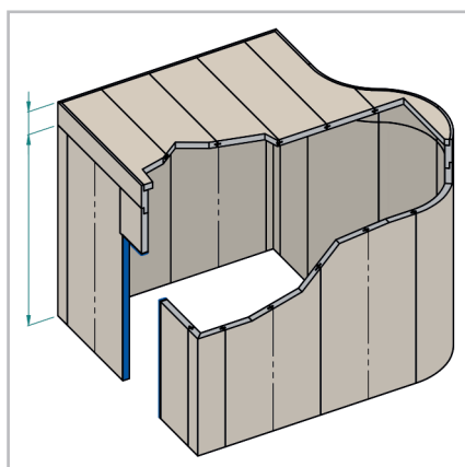
Flexibele wandhoogte: hogere wanden mogelijk door wandverhoging
