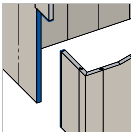
FIX-PRO-MAK 80 mm, rondom aan 3 zijden van de deuropening
