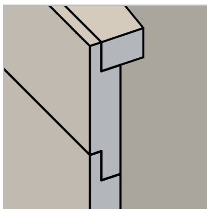
Wandverhoging en dakoplegging met trapspanning
